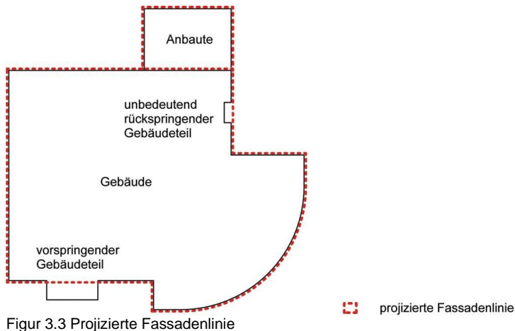
Figur 3.3 Projizierte Fassadenlinie
