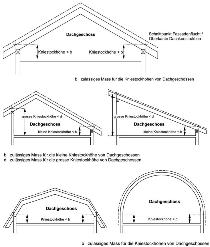
Figur 6.3 Dachgeschosse
